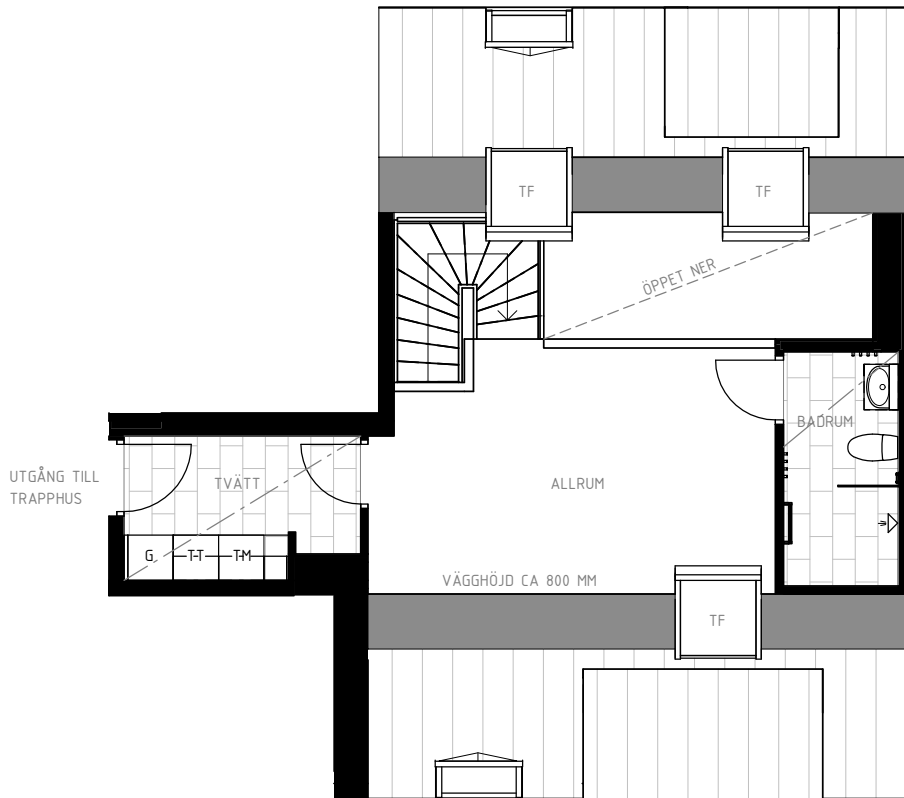
OVANVÅNING (PLAN 7)
