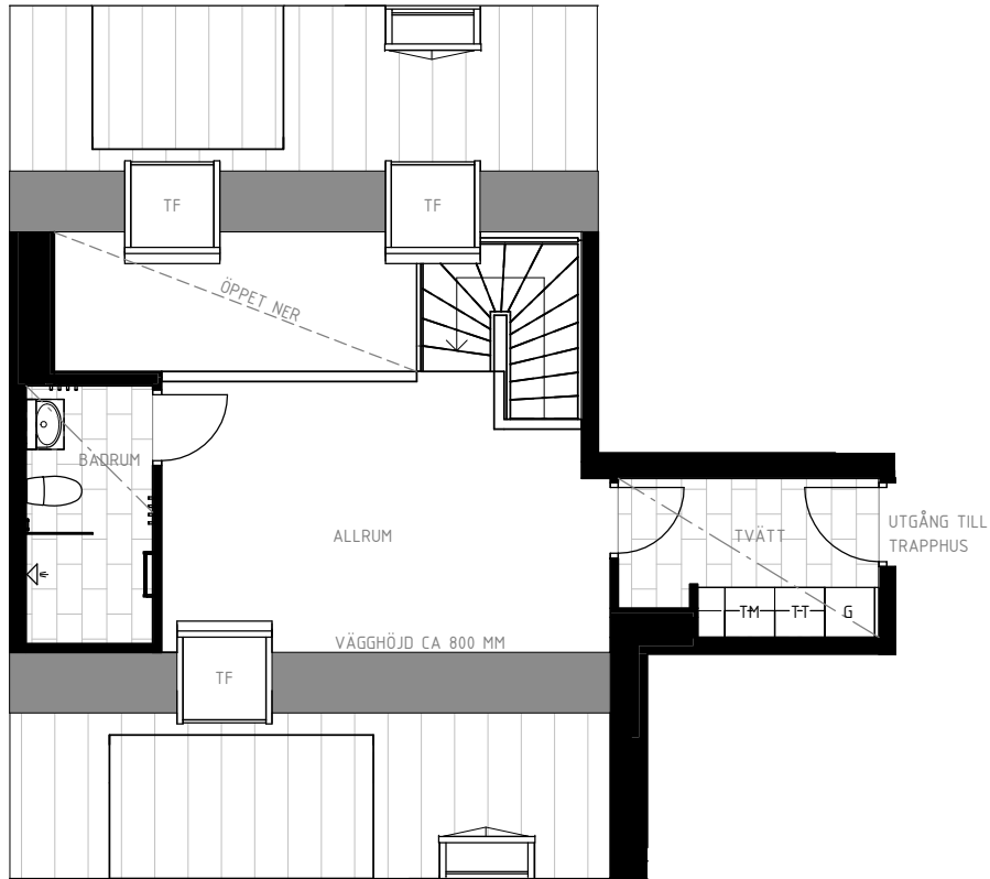
OVANVÅNING (PLAN 7)
