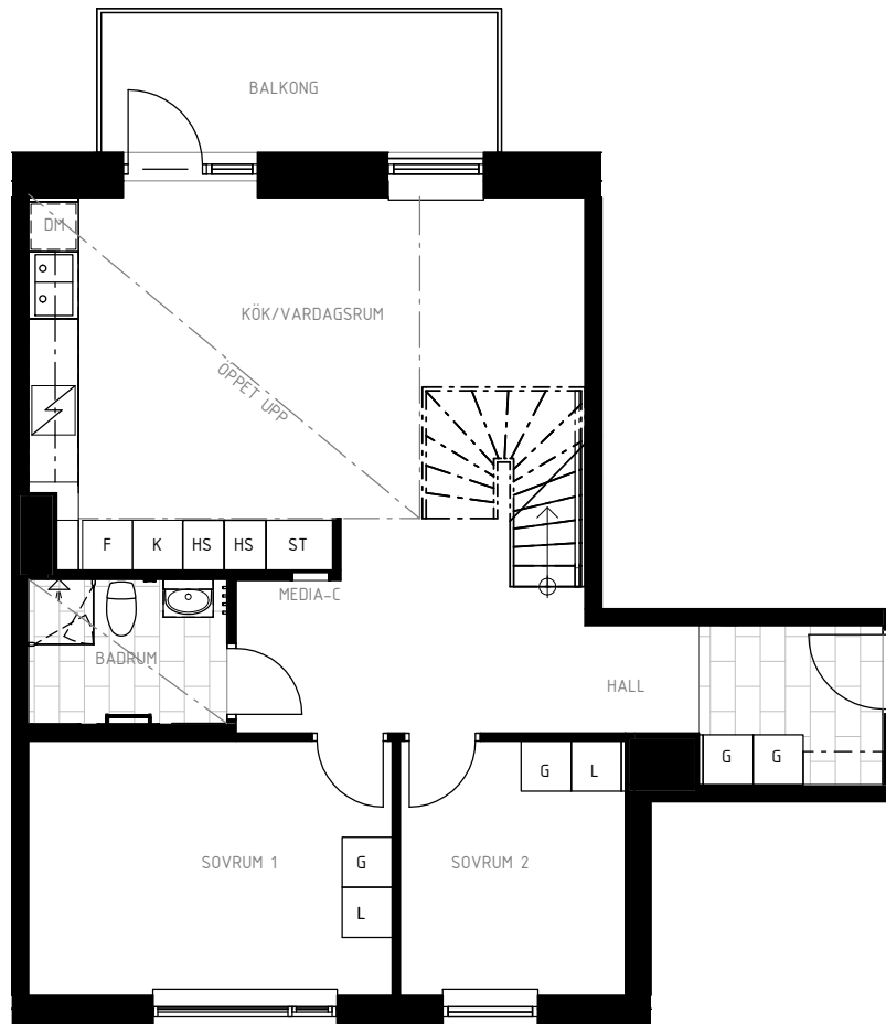
NEDERVÅNING (PLAN 6)
