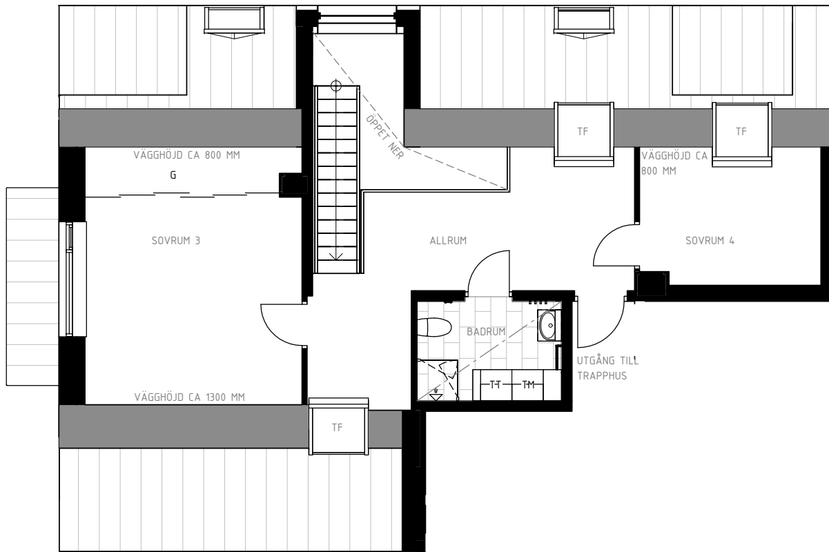
OVANVÅNING (PLAN 7)
